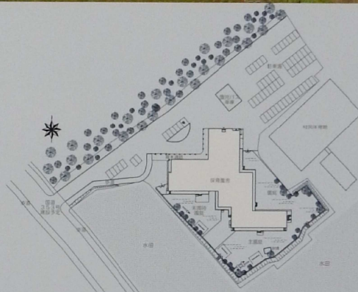
配置図 1:1000
