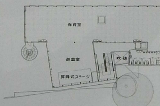
2階平面
