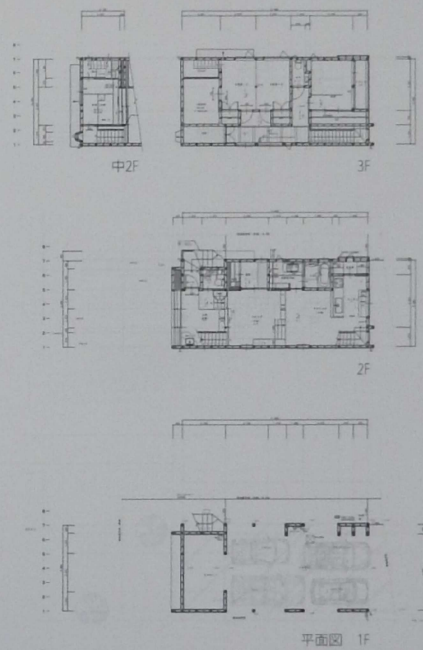
スクリーン(障子)を可変することで、アクティビティに合わせた距離感(パブリック性とプライバシー性の伸縮)を自在にコントロールできる
